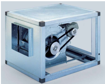
Ιμαντοκίνητο εντός κιβωτίου fan section
